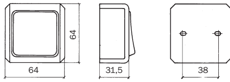
AUFPUTZ-Wippschalter und -taster mit zugehöriger Bodenplatte aus selbstverlöschendem Material.
