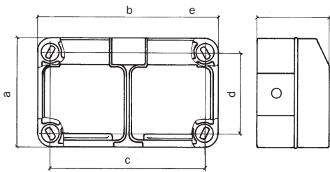
SCHUKO®-Doppel-Steckdose
