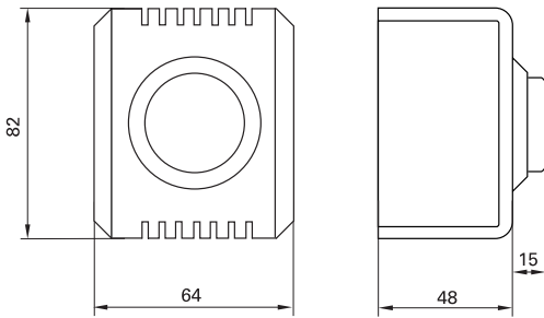
AUFPUTZ-Dimmer Art.-Nr. 5734.., 5716..
