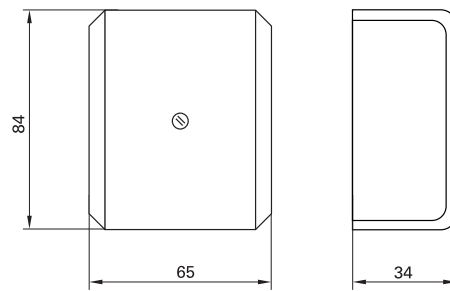
AUFPUTZ-Abzweigdose Art.-Nr. 5230..
