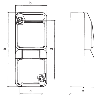
Kombination SCHUKO®- Steckdose / Wechselschalter
