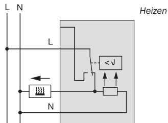
Raumtemperaturregler-Einsatz mit Wechslerkontakt Art.-Nr. 5364..
