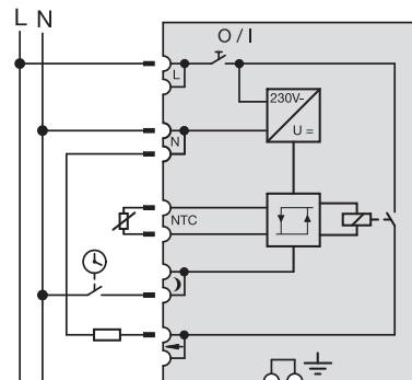
Fußbodentemperaturregler-Einsatz mit Schalter Art.-Nr. 537100
