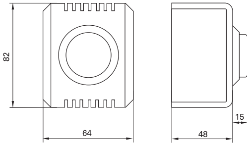
AUFPUTZ-Dimmer Art.-Nr. 5734.., 5716..
