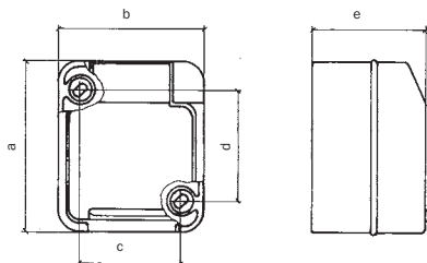
1fach SCHUKO-Steckdose
