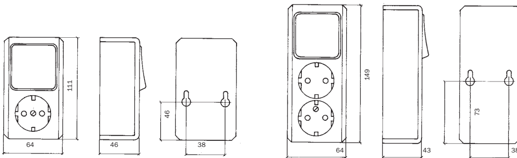
AUFPUTZ-Kombination SCHUKO-Steckdose / Wechselschalter mit zugehöriger Bodenplatte aus selbstverlöschendem Material.
