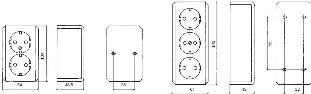
AUFPUTZ-SCHUKO-Doppel-Steckdose mit zugehöriger Bodenplatte aus selbstverlöschendem Material.
