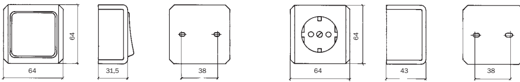
AUFPUTZ-Wippschalter und -taster mit zugehöriger Bodenplatte aus selbstverlöschendem Material.
