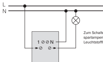
Relais-Universal-Einsatz 575897
