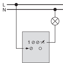
Superdimmer
