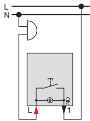
Taster mit Orientierungslicht, Schließer MEG3160-0000
