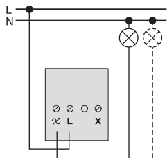
Drehdimmer mit Druck-Ausschalter MEG5131-0000
