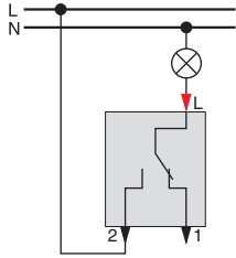
Aus-/Wechselschalter
