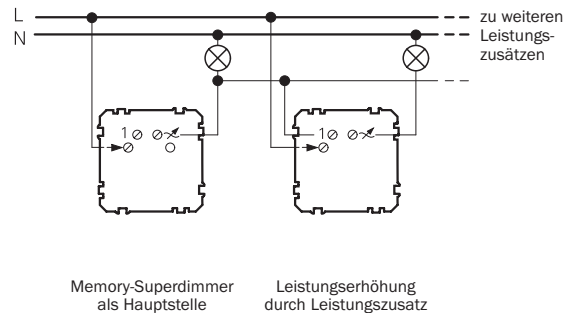
Memory-Superdimmer mit Leistungszusatz
