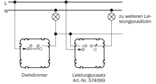
Glühlampen-Drehdimmer Ein-/Ausschaltung mit Leistungszusatz
