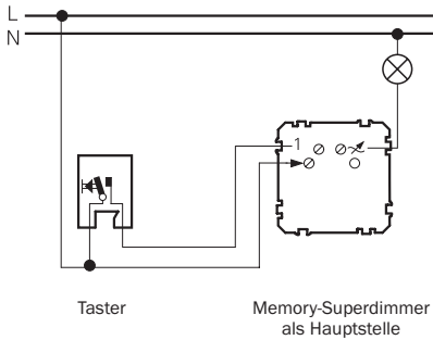
Dimmbare Wechselschaltung mit Taster
