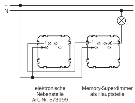
Dimmbare Wechselschaltung mit Nebenstelle
