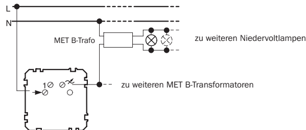
ET-Memory-Superdimmer Art.-Nr. 5778.. mit Sensor- oder TELE-Tastfläche
