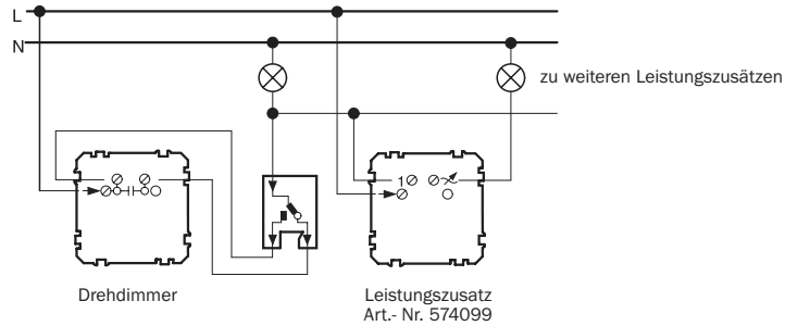
Glühlampen-Drehdimmer Wechselschaltung mit Leistungszusatz
