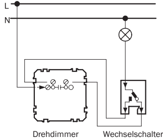
Glühlampen-Drehdimmer Wechselschaltung
