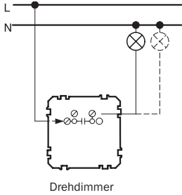
Glühlampen-Drehdimmer Ein-/Ausschaltung
