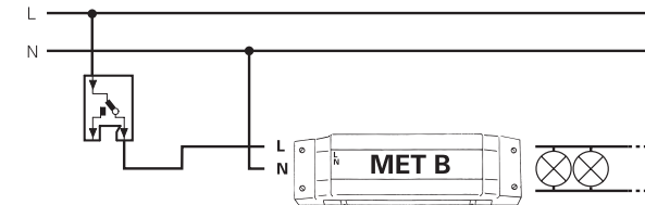
Wechselschalter
