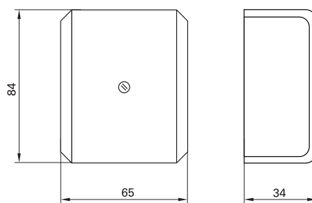
AUFPUTZ-Abzweigdose Art.-Nr. 5230..
