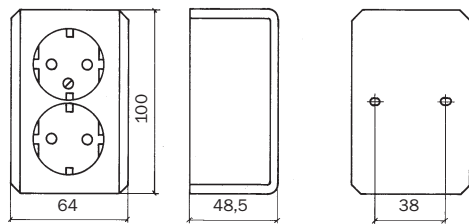
AUFPUTZ-SCHUKO®-Doppel-Steckdose mit zugehöriger Bodenplatte aus selbstverlöschendem Material.
