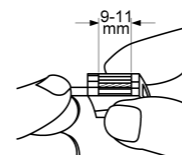
Bild 6: Abisolierlänge
