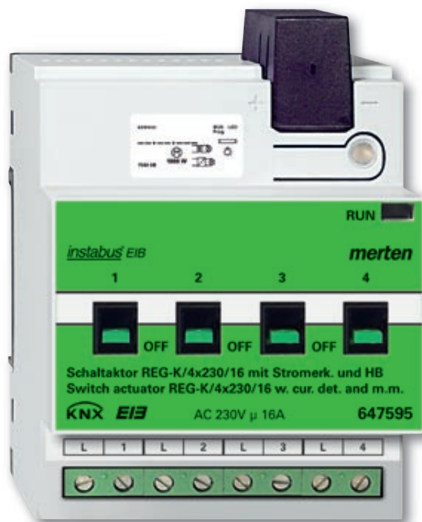
KNX-schakelactor REG-K/4x230/16 met handbediening en stroomdetectie
